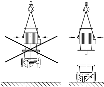
Рис. 8: Транспортировка электродвигателя
