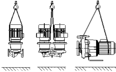
Рис. 7: Транспортировка насоса
